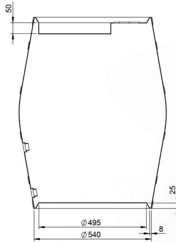
SECTION A-A
